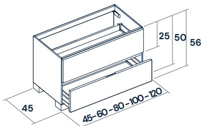
Low 2 floor drawers Bas 2 tiroirs au sol Bajo 2 cajones a suelo
