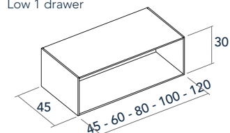
Bajo abierto h30 Bas ouvert h30 Open low h30
