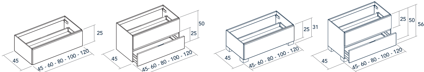
Bajo 1 cajón Bas 1 tiroir Low 1 drawer
