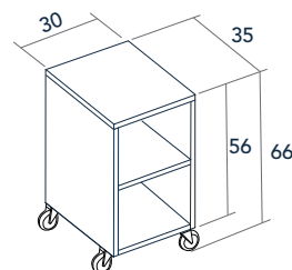
Carro con estante Chariot avec étagère Cart with shelf
