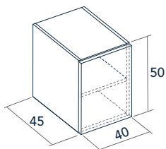
Bajo con puerta Bas avec porte Low with door
